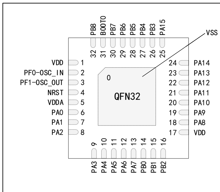
图 5 APM32E030x8 系列 QFN32 引脚分布图
