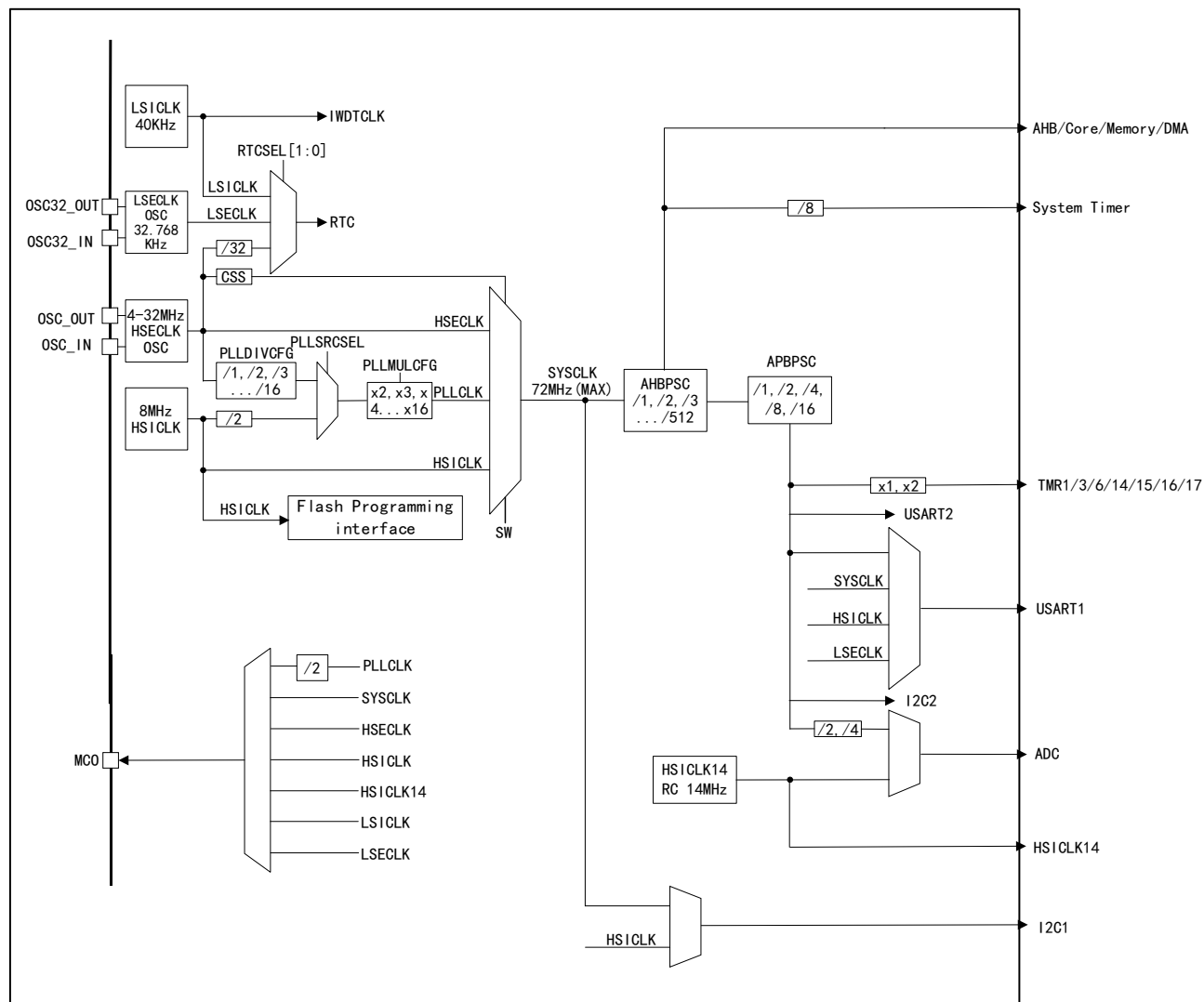
图 10 APM32E030x8 时钟树
