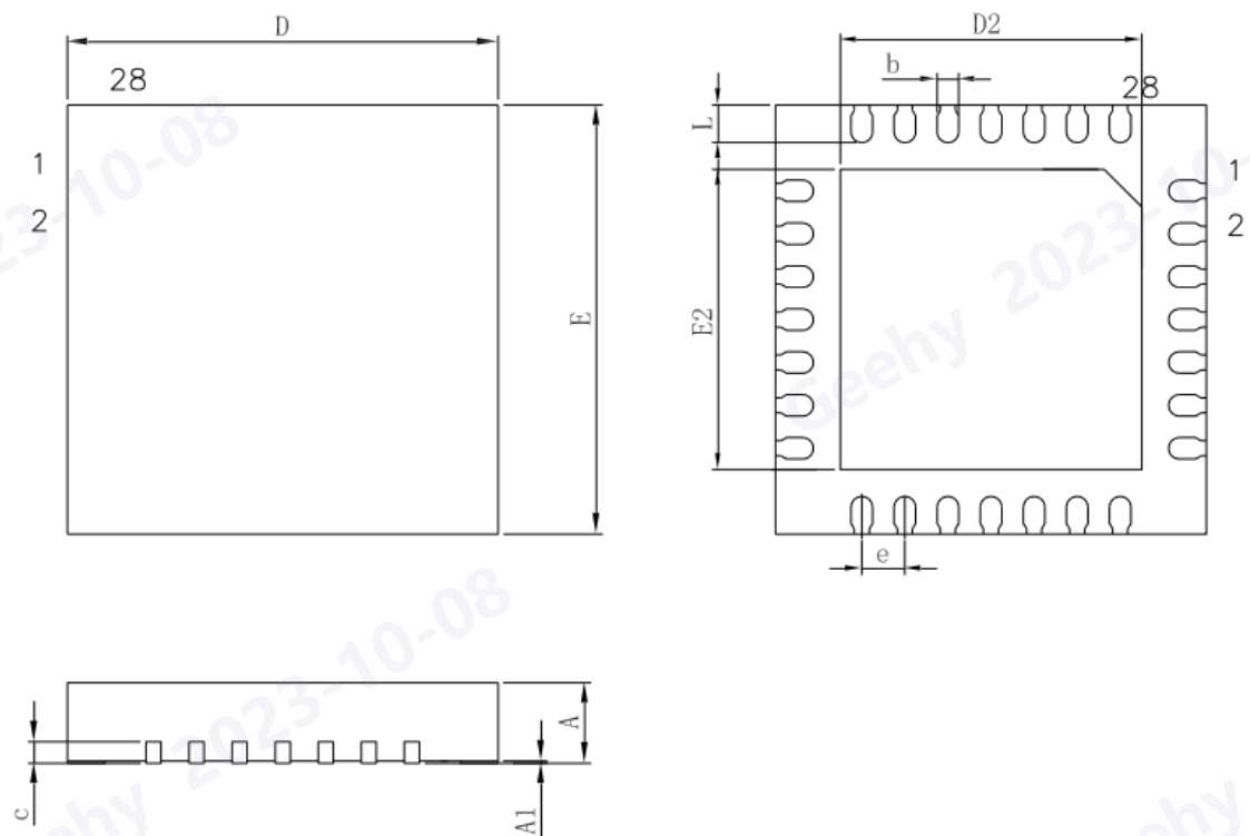
图 35 QFN28 封装图
