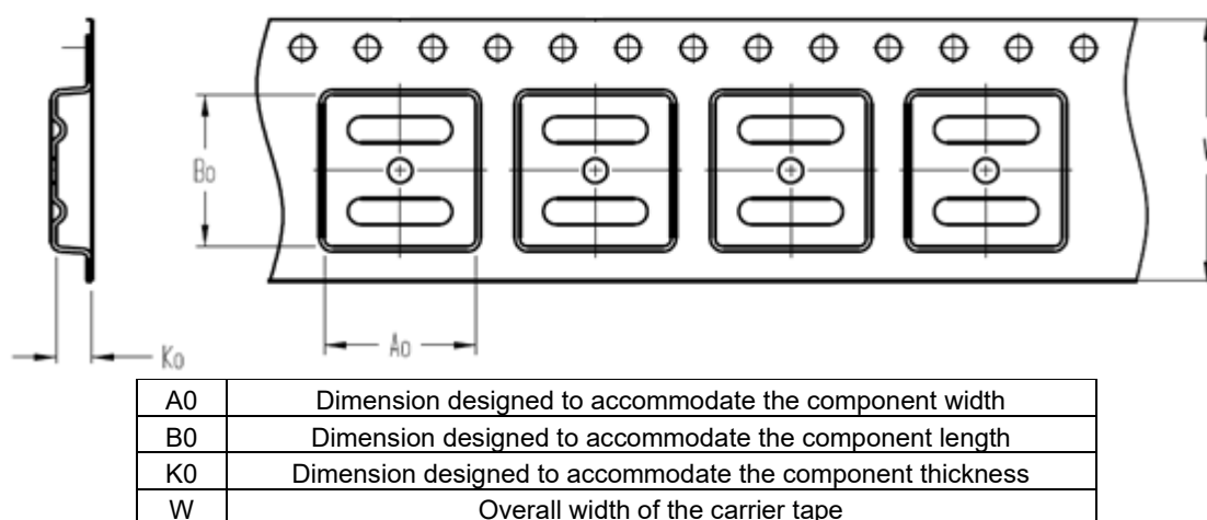
图 41 带状包装规格图
