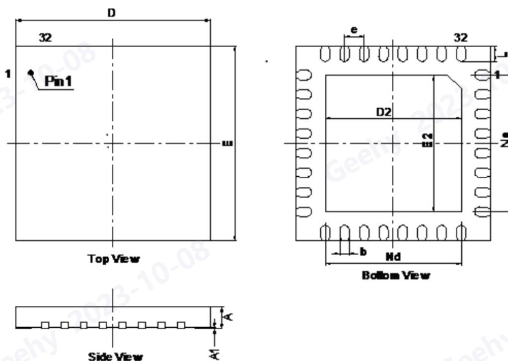
图 32 QFN32 封装图
